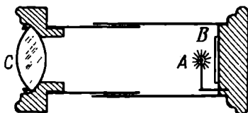
Fig. 211. A spinthariscopes
