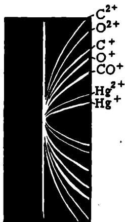
Fig. 217. Ion parabolas
