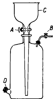
Fig. 14. A gas holder
