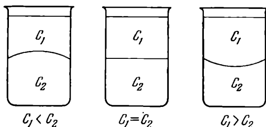
Fig. 81. Osmosis
